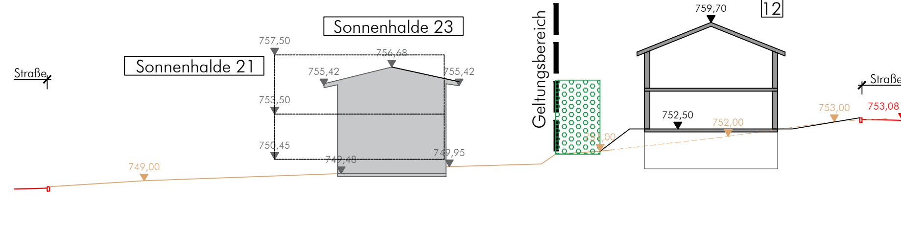
Schnittachse VII 740,00 NHN
