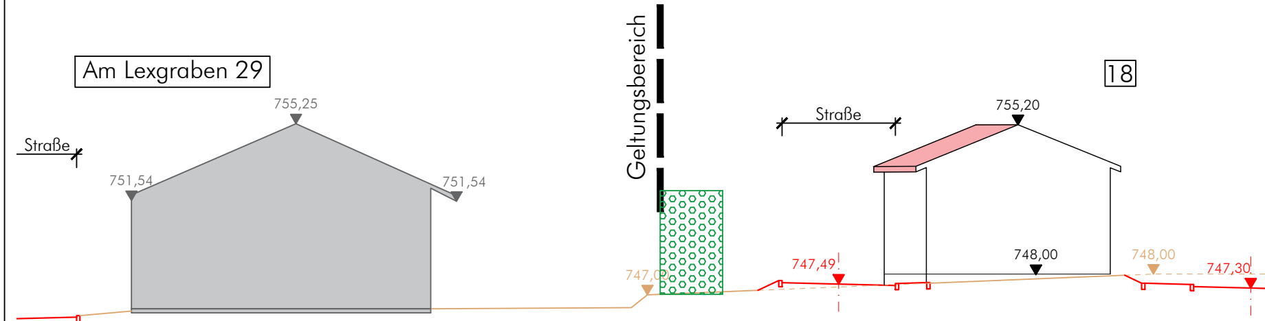
Schnittachse I 740,00 NHN
