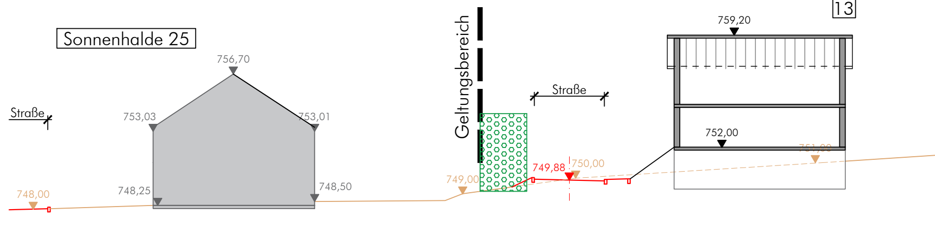
Schnittachse VI 740,00 NHN
