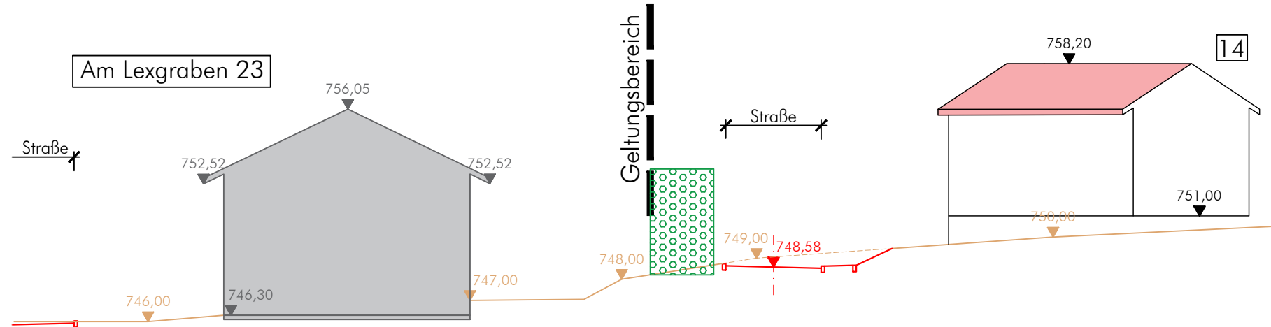
Schnittachse IV 740,00 NHN
