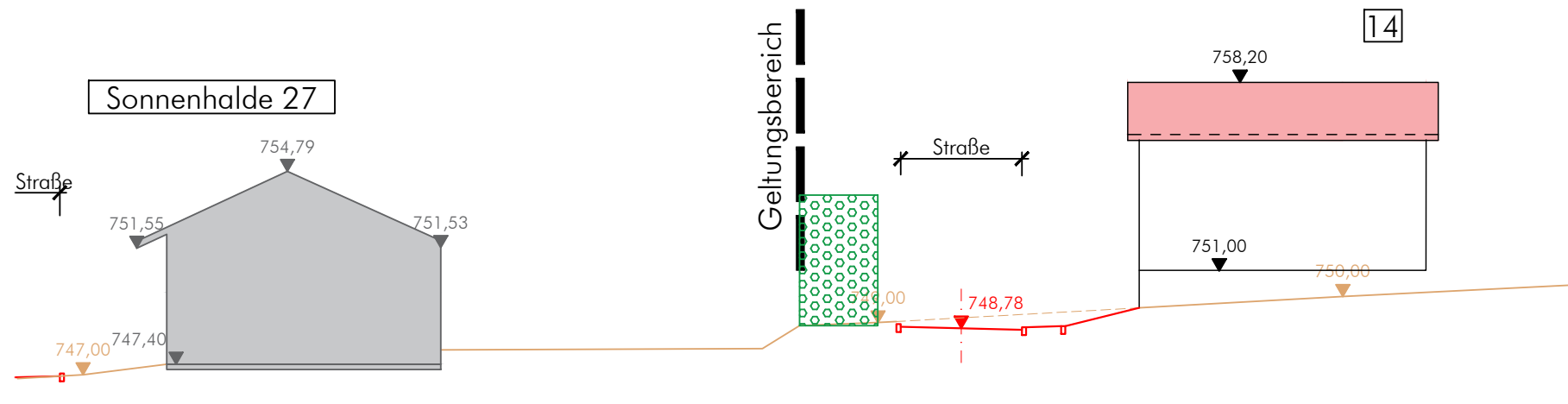
Schnittachse V 740,00 NHN
