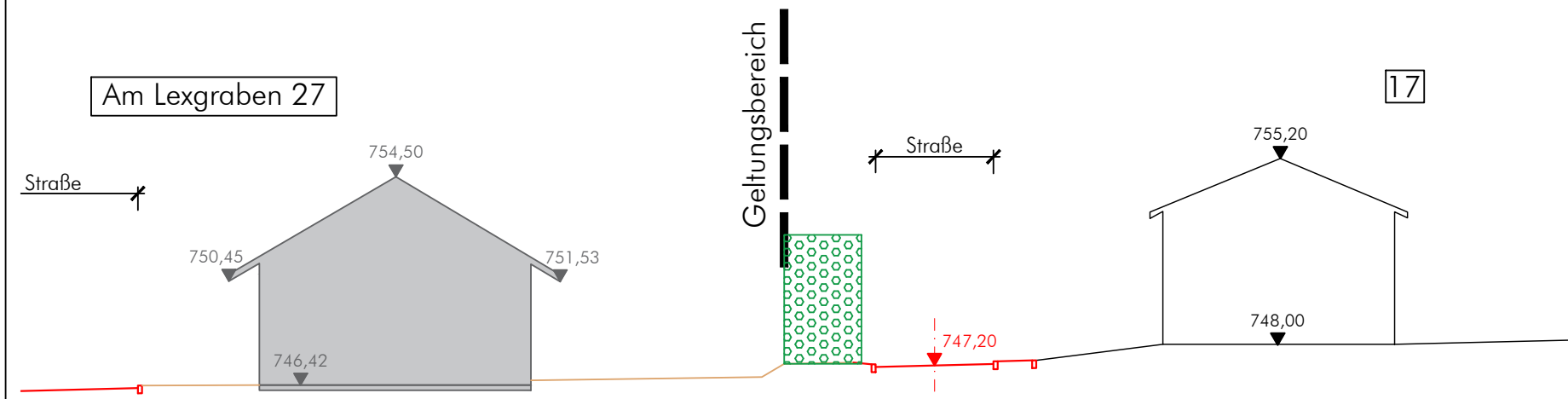
Schnittachse II 740,00 NHN
