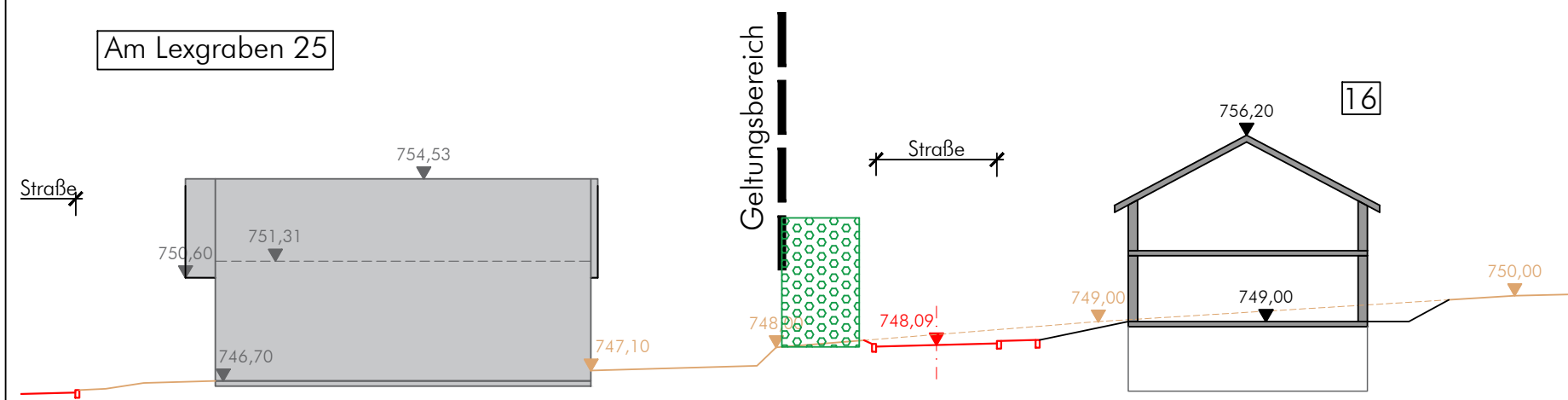
Schnittachse III 740,00 NHN
